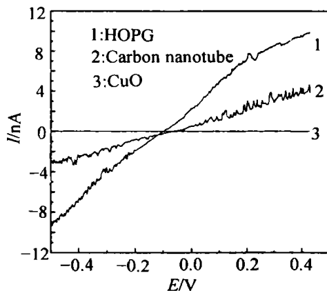
图 7 HOPG/CuO 基底上碳纳米管的 I-E 曲线
