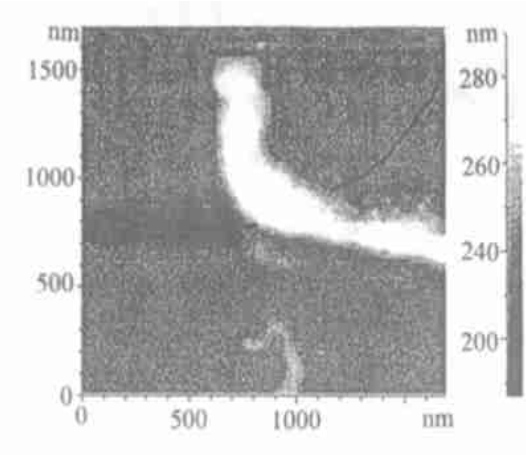
图 3 Au/ CuO 基底上表面碳纳米管的形貌(扫描范围:1.7 \mu\text{m} \times 1.7 \mu\text{m} )
